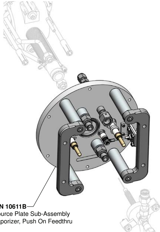
P/N 10260V
